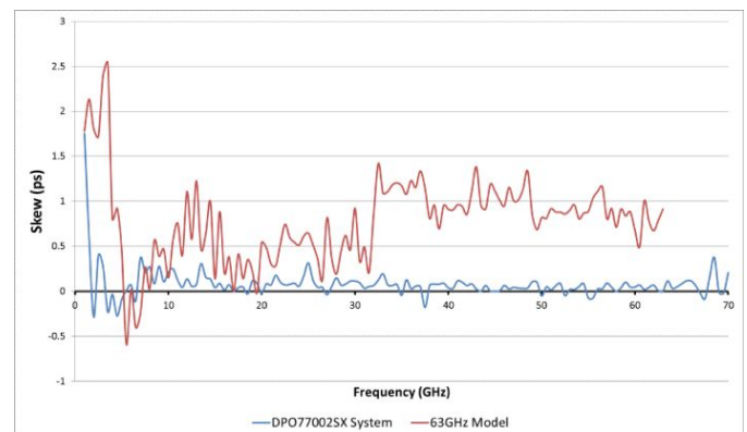
Сравнение зависимости фазового сдвига между двумя каналами от частоты в двухприборной системе DPO77002SX и двухканальной одноприборной системе с полосой пропускания 63 ГГц другого производителя.
